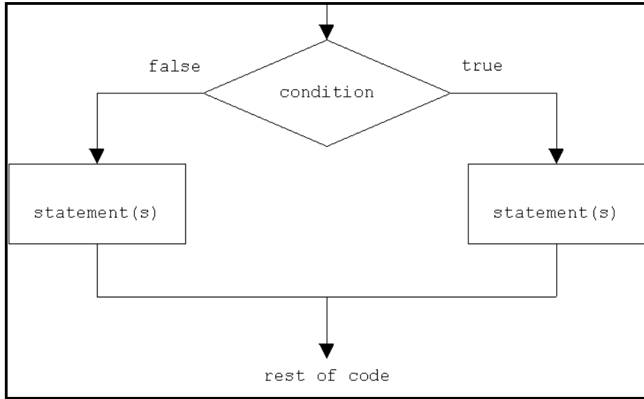
চিত্র : (৬.৬.২) if else ফ্লো-চার্ট ।
